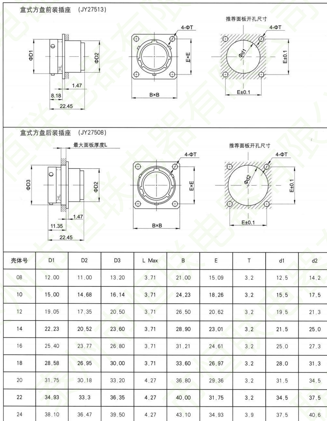
【盒式方盘插座 JY27513 / JY27508】
