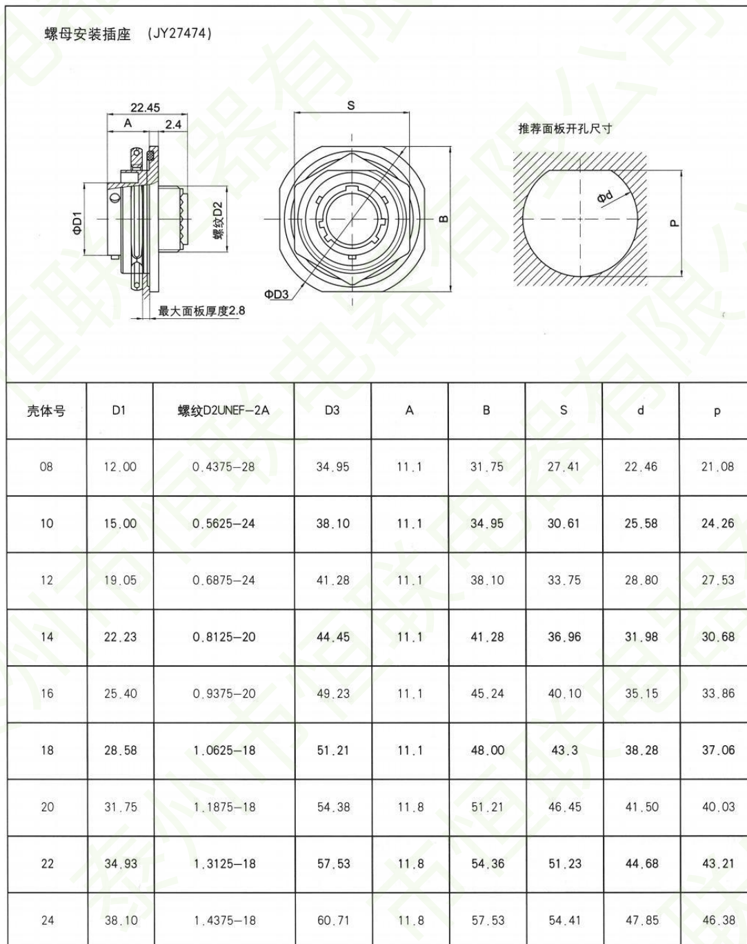
【螺母安装插座 JY27474】
