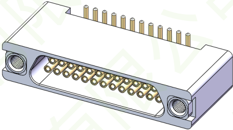
产品外形尺寸图
