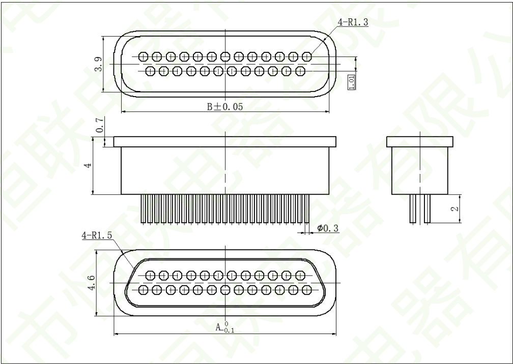
产品外形尺寸图
