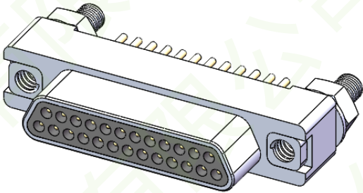
产品外形尺寸图
