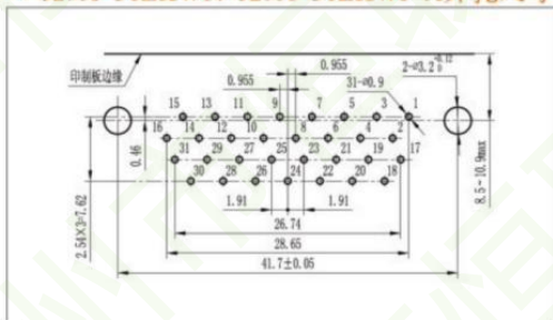
▼ J29A-31ZKWI、J29A-31ZKWI-A开孔尺寸
