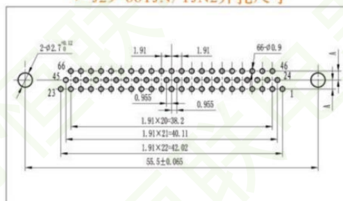
▼ J29-66TJN/TJN2开孔尺寸
