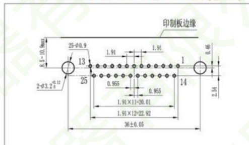
▼ J29A-25ZKW、J29-25ZKW-A开孔尺寸
