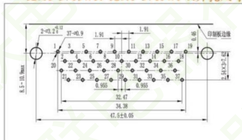
▼ J29A-37TJWI、J29A-37TJWI-A开孔尺寸
