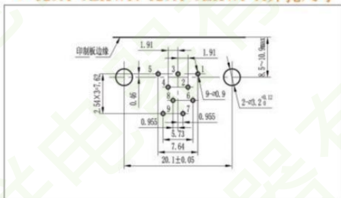
▼ J29A-9ZKWI、J29A-9ZKWI-A开孔尺寸
