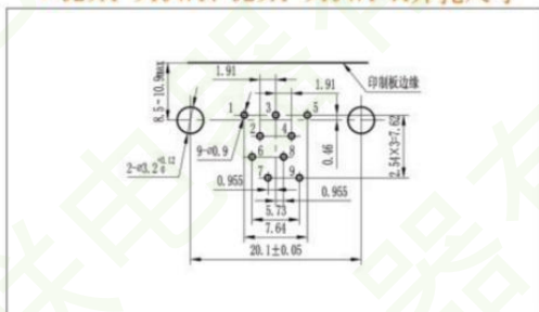
▼ J29A-9TJWI、J29A-9TJWI-A开孔尺寸
