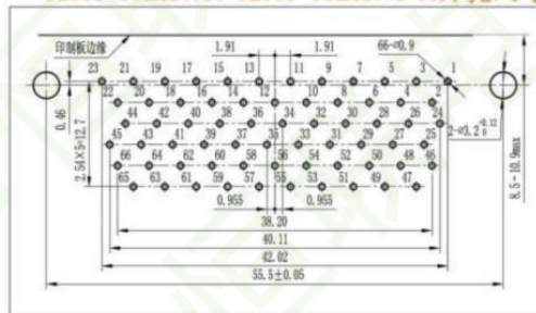
▼ J29A-66ZKWI、J29A-66ZKWI-A开孔尺寸
