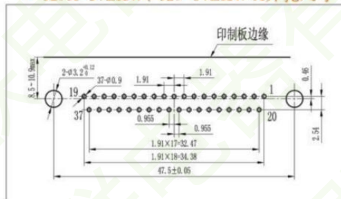
▼ J29A-37ZKW、J29-37ZKW-A开孔尺寸
