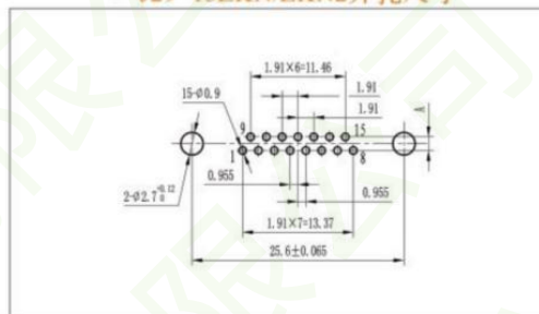
▼ J29-25ZKN/ZKN2开孔尺寸
