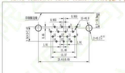
▼ J29A-15ZKWI、J29A-15ZKWI-A开孔尺寸
