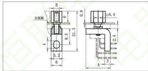
▼ 外形尺寸图
