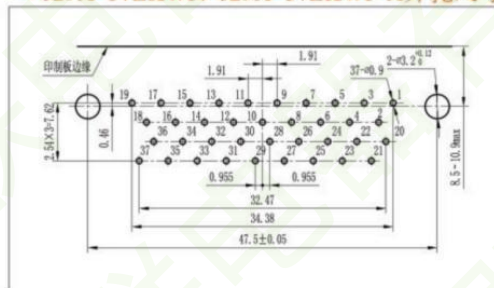
▼ J29A-37ZKWI、J29A-37ZKWI-A开孔尺寸
