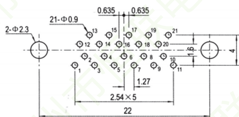
J30-21ZKN
