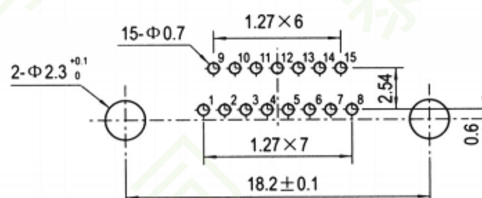
J30-15ZKW-J
