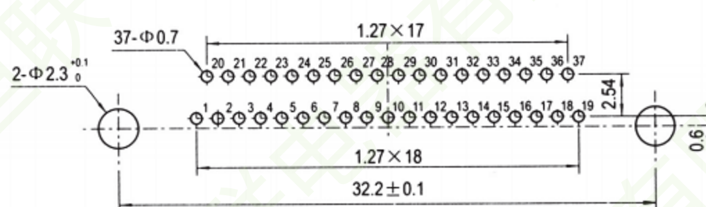
J30-37ZKW-J
