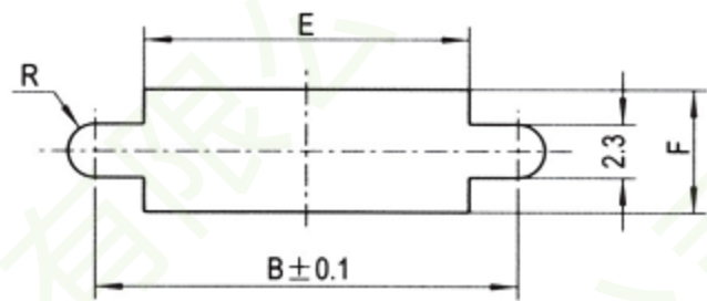
J30插座板前安装开孔尺寸
