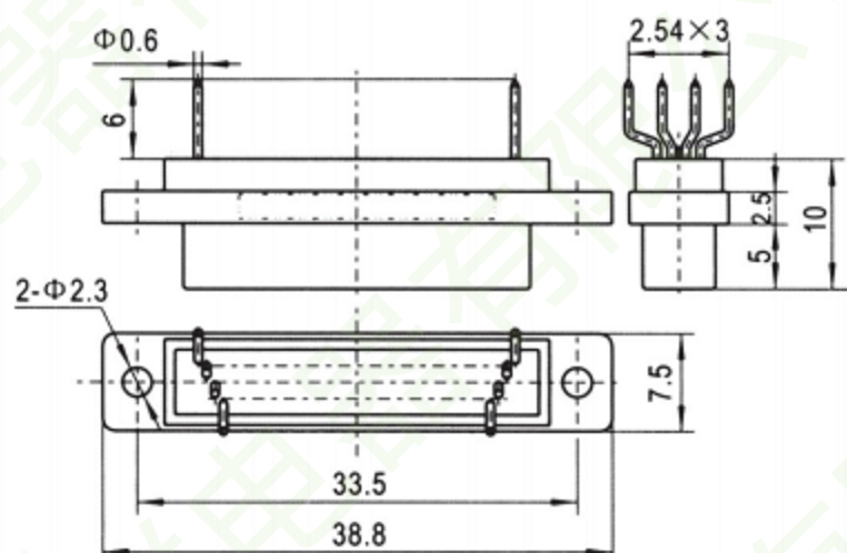
J30-74TJN-J
