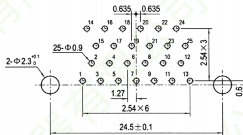
J30-25ZKW
