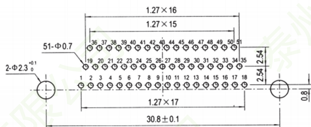
J30-51ZKW-J
