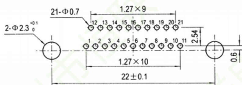
J30-21ZKW-J
