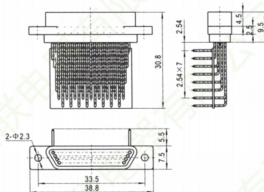
J30-74ZKW
