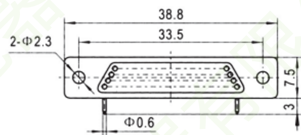
J30-74TJW-J
