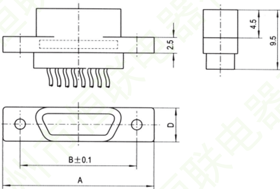
J30-ZK
