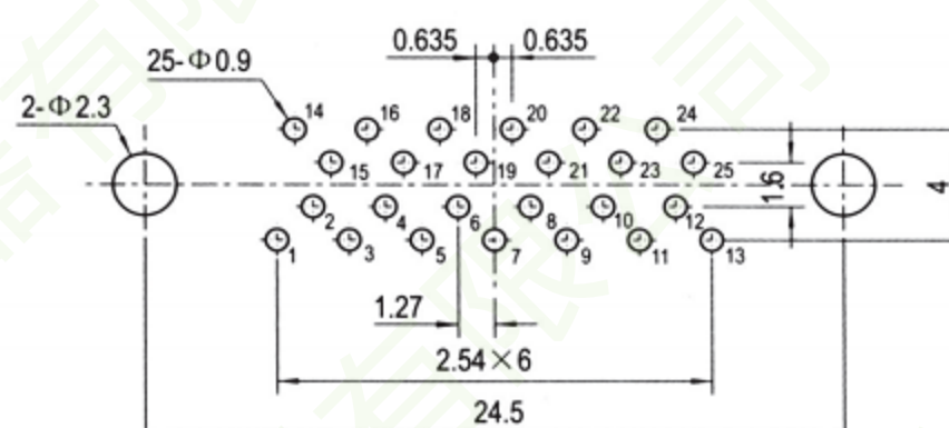
J30-25ZKN
