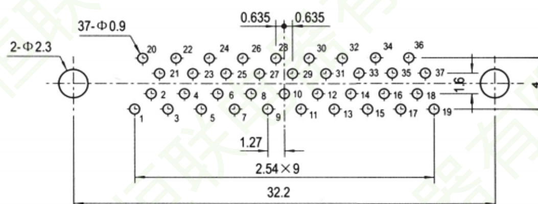
J30-37ZKN
