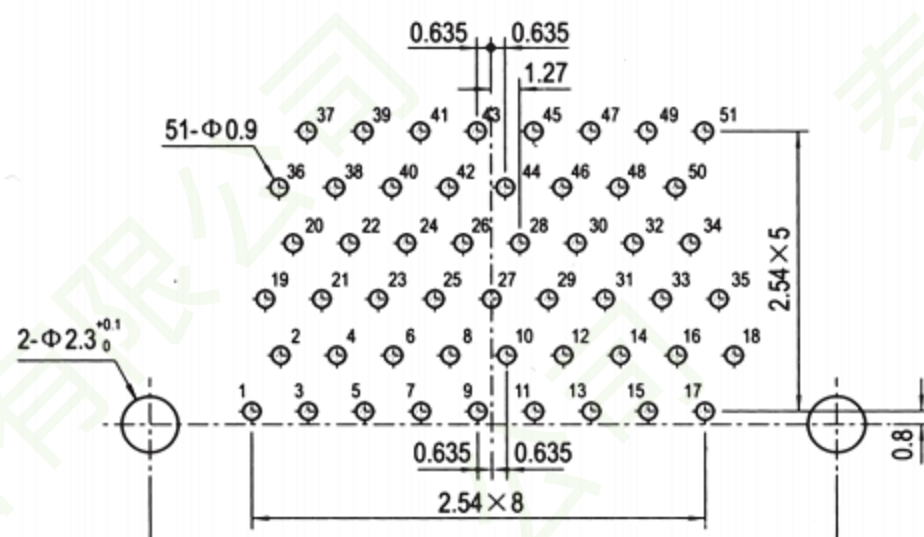
J30-51ZKW
