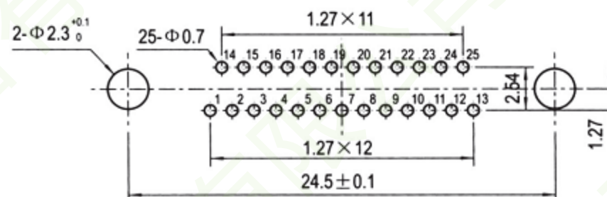
J30-25ZKN-J
