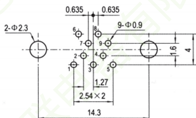
J30-9ZKN
