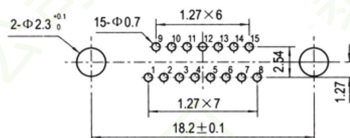
J30-15ZKN-J
