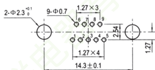
J30-9ZKN-J
