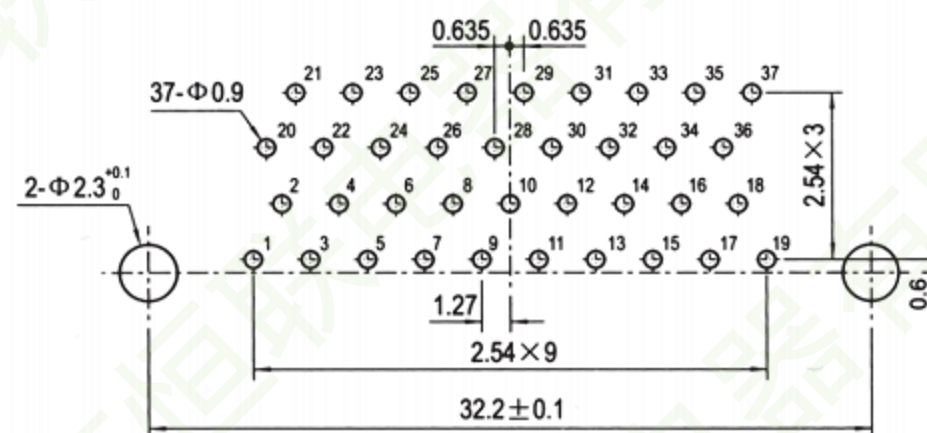
J30-37ZKW
