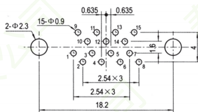
J30-15ZKN
