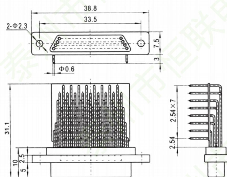
J30-74TJW
