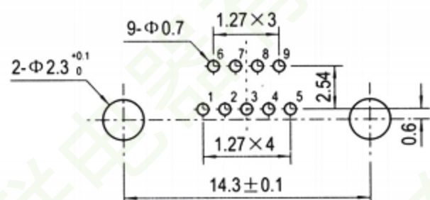
J30-9ZKW-J
