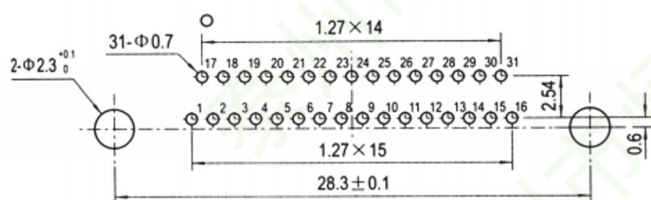
J30-31ZKW-J
