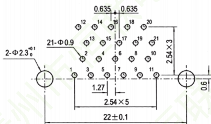
J30-21ZKW
