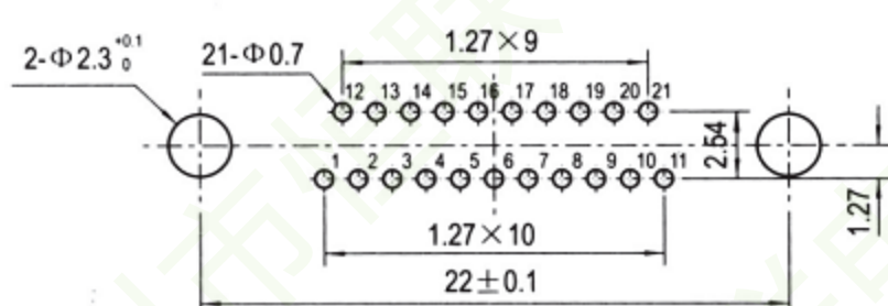
J30-21ZKN-J
