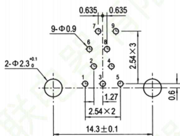
J30-9ZKW
