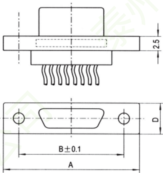
J30-TJ
