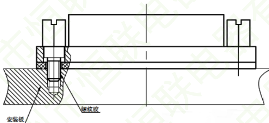
安装示意图
