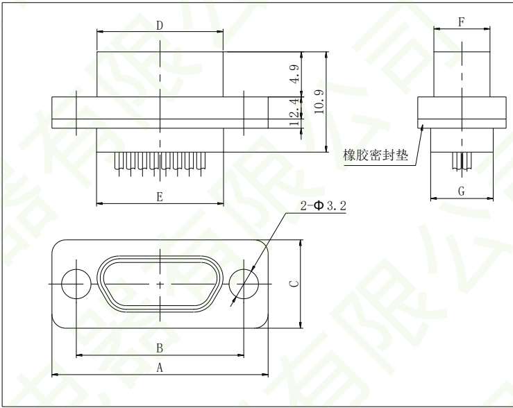
J30JY-□ZK
