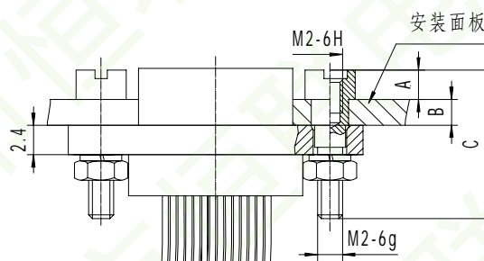
外形尺寸图
