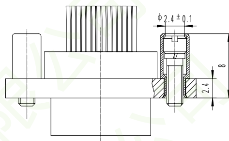
外形尺寸图
