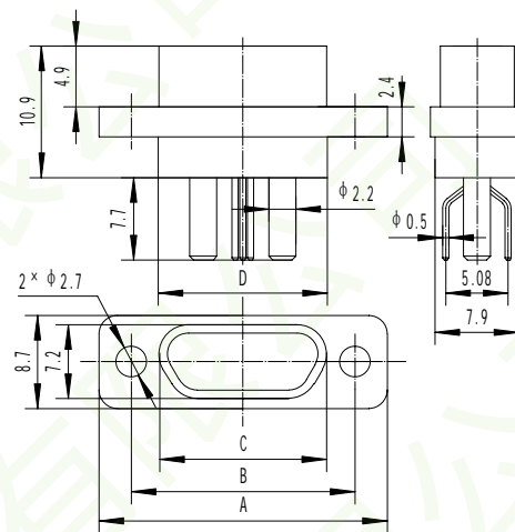
产品外形尺寸图
