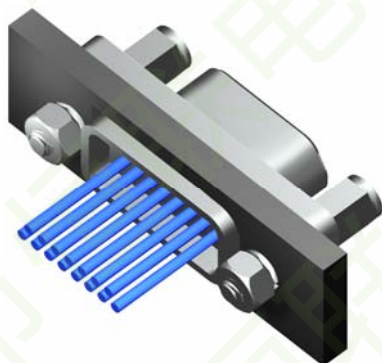
组装示意图
