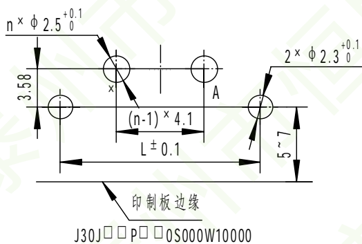
J30J 系列弯式印制板混装产品推荐印制板开孔尺寸
