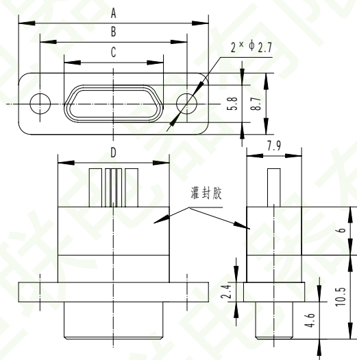
产品外形尺寸图
