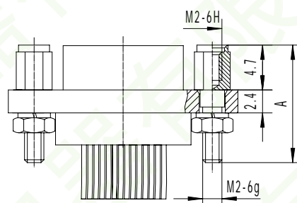
外形尺寸图
