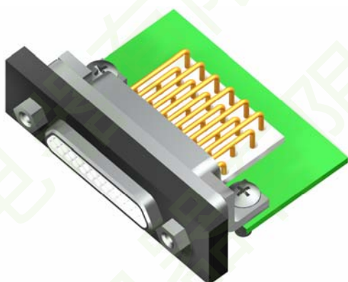
组装示意图
