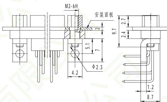
外形尺寸图
