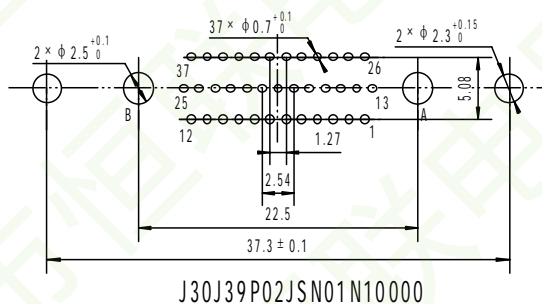
J30J 系列弯式印制板混装产品推荐印制板开孔尺寸
