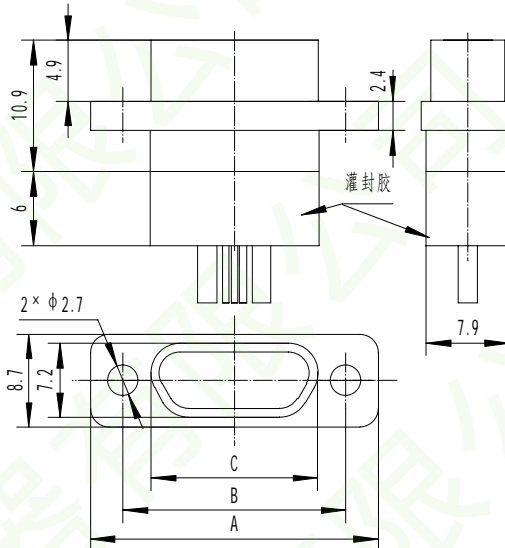
产品外形尺寸图
