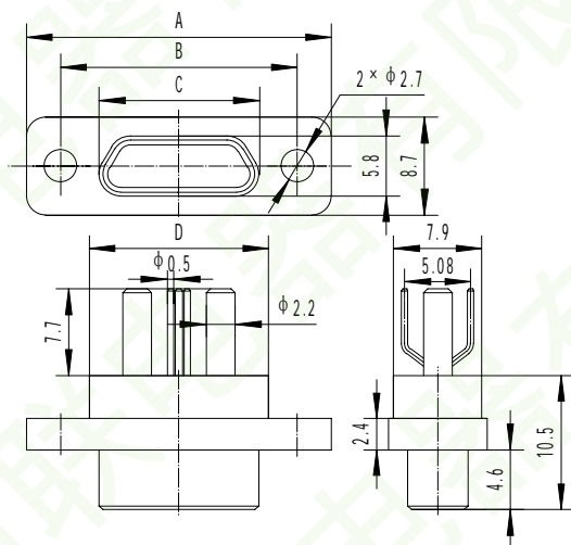
产品外形尺寸图
