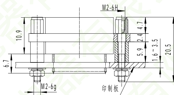
外形尺寸图
