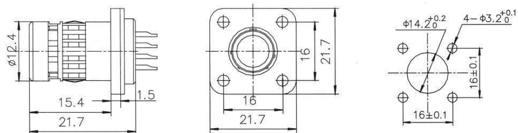
安装开孔尺寸
