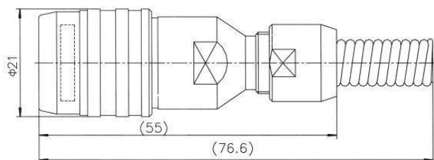
TL24H26×10××J03A（φ5）插头
