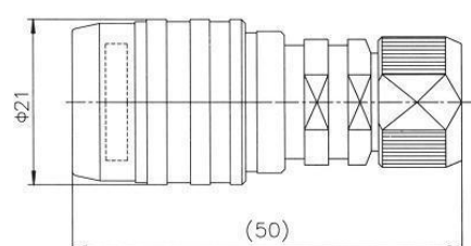
TL24H26×10××J03A（φ5）插头
