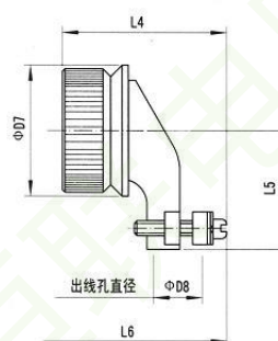
弯式电缆夹
