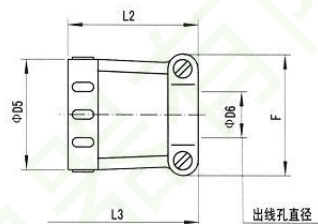
直式电缆夹
