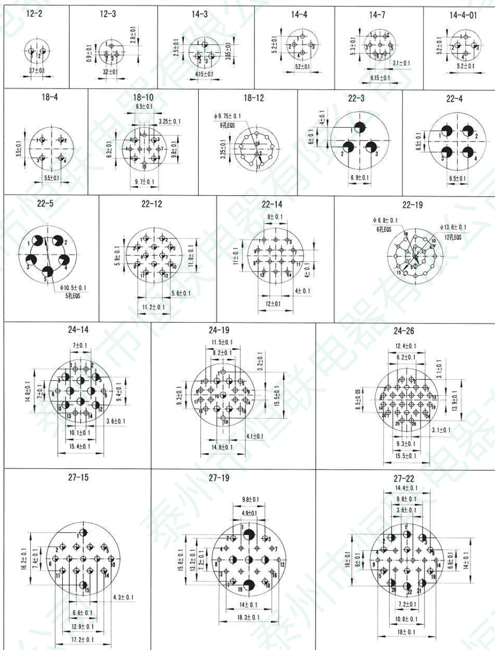
XCEB印制板布线建议尺寸 (装针绝缘体印字面)
