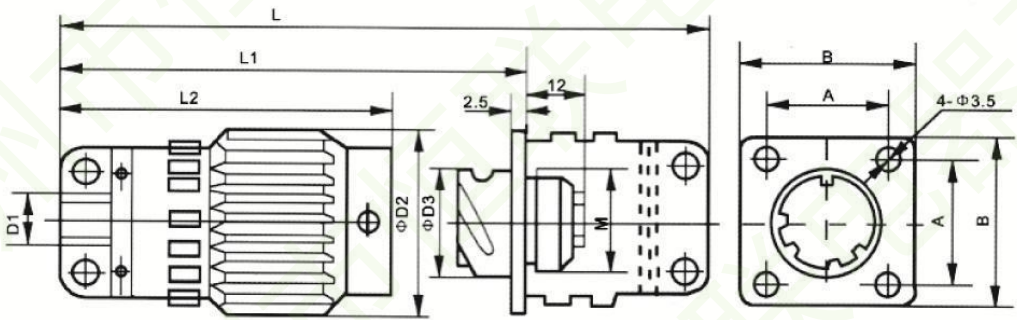
Y2圆型电连接器外形安装尺寸
