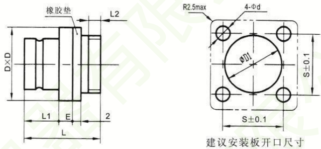
建议安装板开口尺寸
