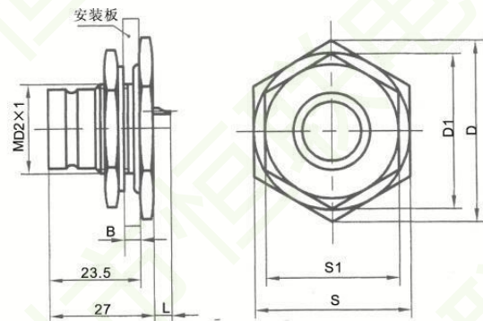
螺母安装(B2)橡胶密封插座
