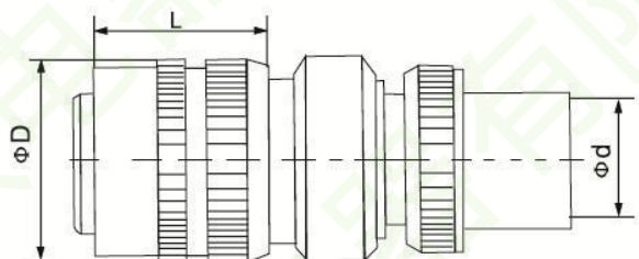
4. 防波抗拉式插头外形尺寸
