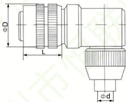
5. 弯头式外形尺寸
