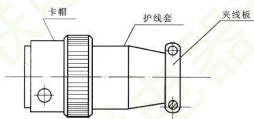
7. 并紧护线式(等同夹线板式)
