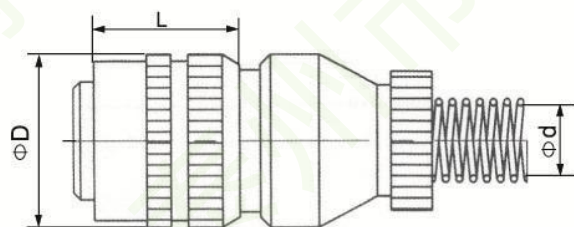
6. 弹簧护线式外形尺寸
