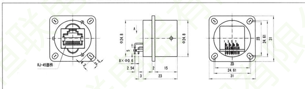
[YW120F01W 卡口连接方盘安装弯式印制板插座]
