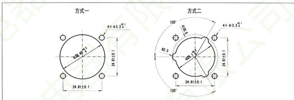
[YW120F01B 卡口连接方盘安装直式印制板插座]
