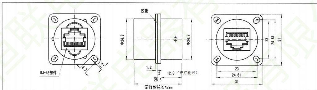
[YW121F01 单卡口连接方盘安装转接插座]
